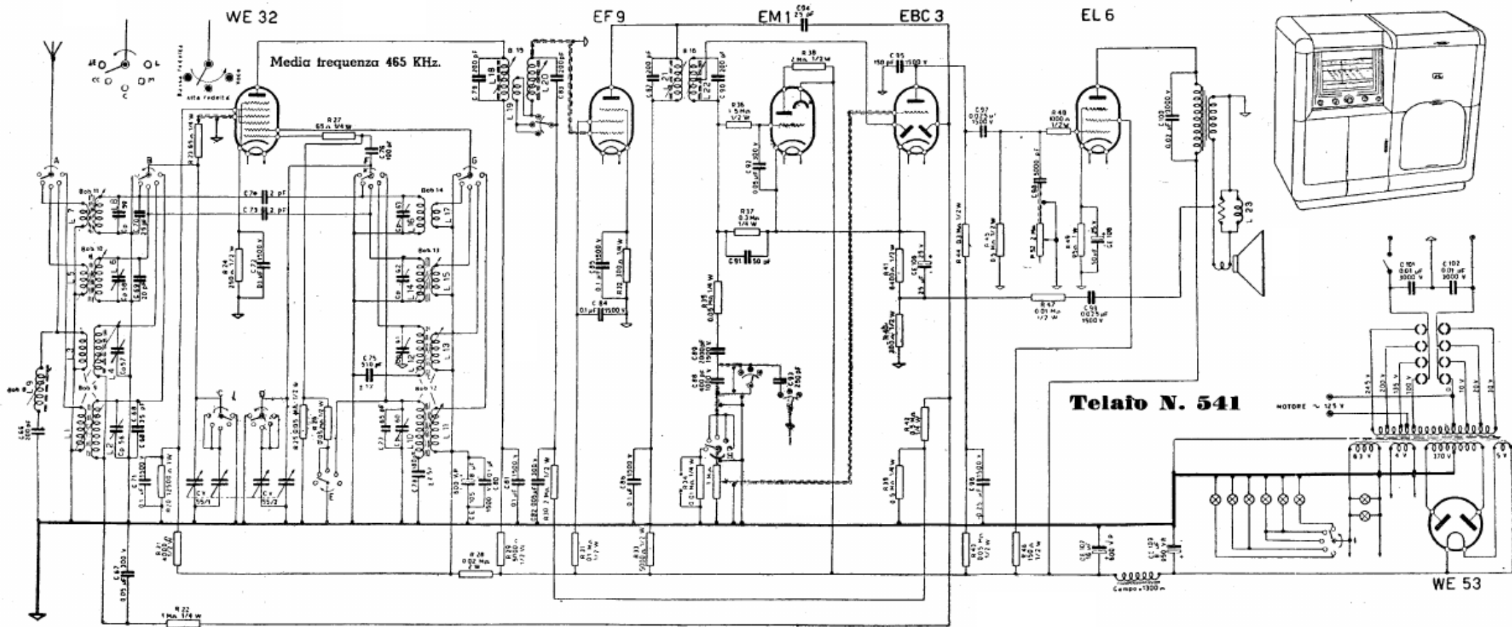
LA VOCE DEL PADRONE. — «Mod. 544». — Produzione 1939-1940. — Media frequenza 465 kHz.
